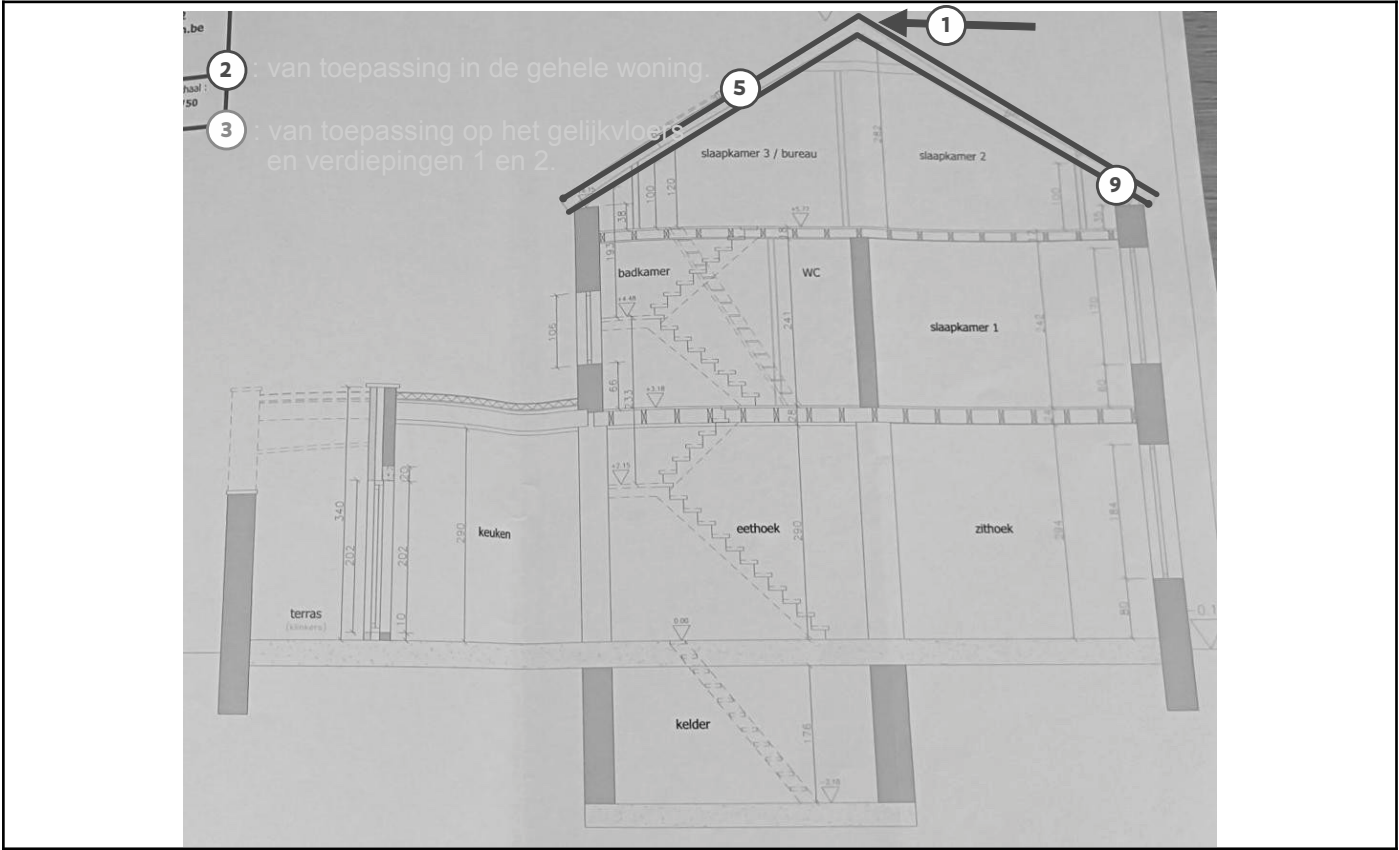
Legende van plan 1.5: Doorsnede
